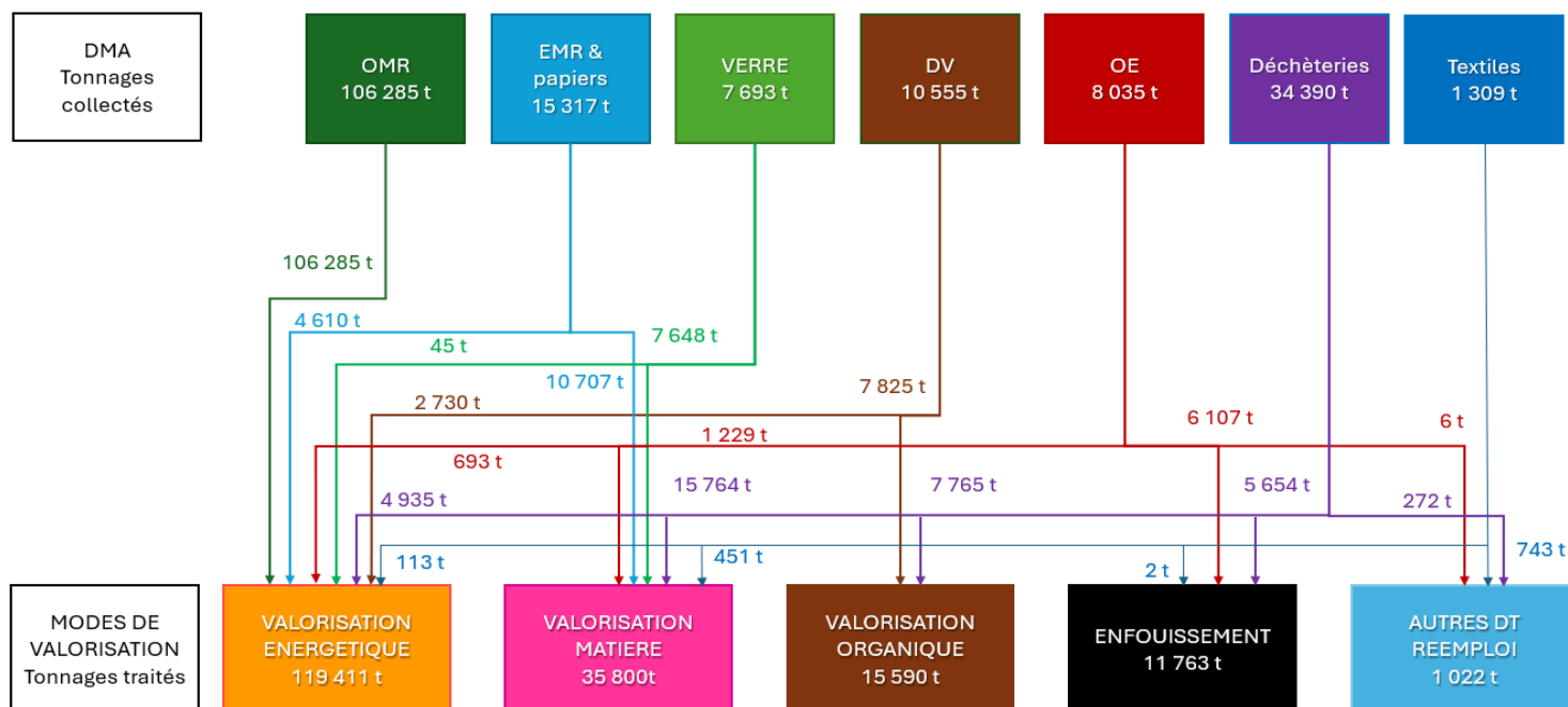
Figure 33 : synoptique des flux collectés et traités par la CU GPS&O
